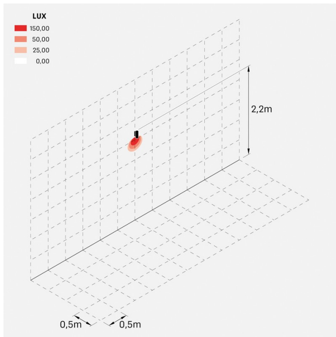
ago_applique_5w_optic_d
